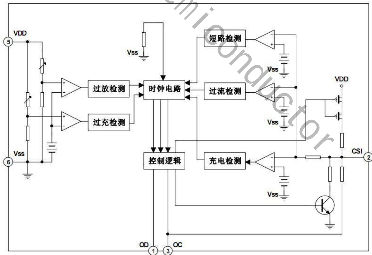
图2 功能框图
